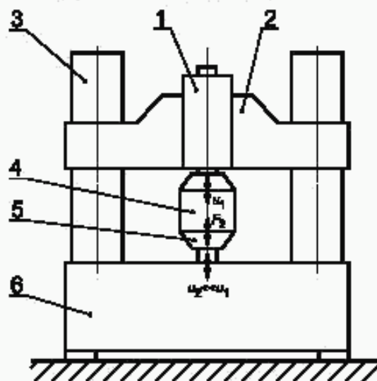
1 — исполнительное устройство гидравлического типа (обеспечивает предварительное статическое нагружение и динамическое возбуждение); 2 — траверсы; 3 — направляющие стойки; 4 — испытуемый виброизолятор; 5 — система измерения силы; 6 — жесткое основание
