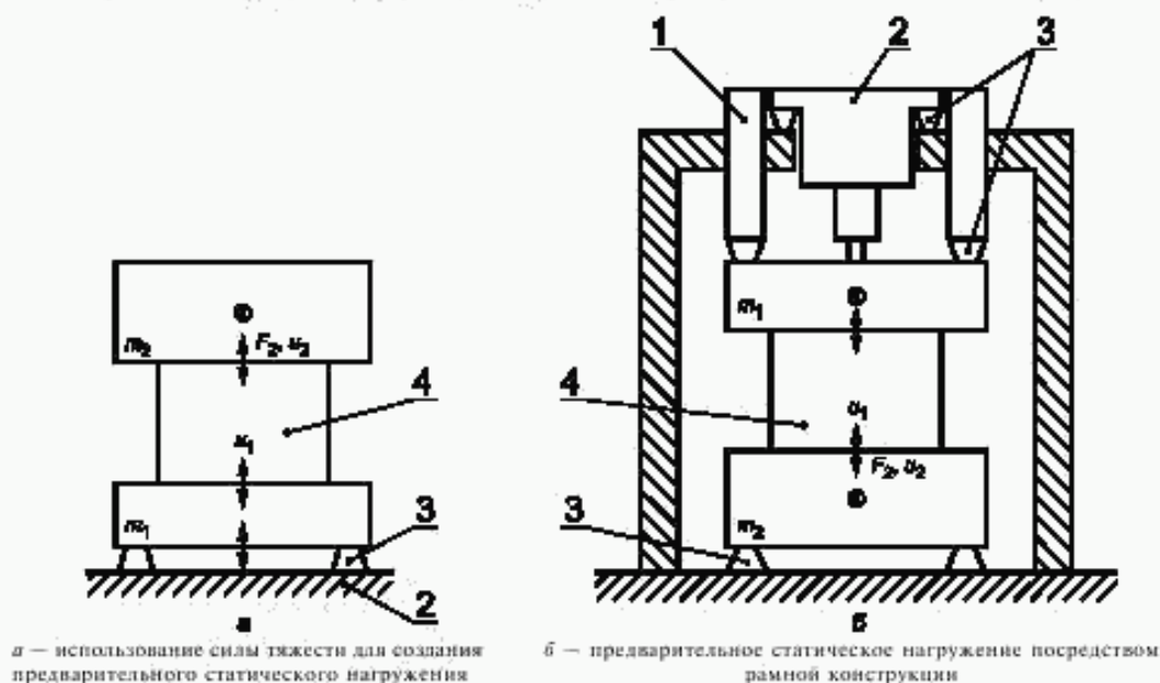
Рисунок 3 — Пример испытательной установки для косвенного метода измерений
