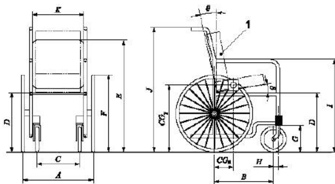
Рисунок D.1 — Критические спецификации MSWC
