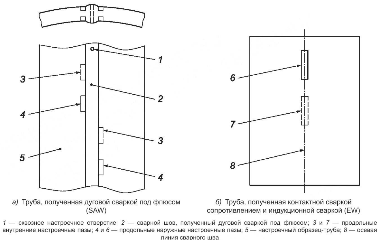
Рисунок 1 — Схема настроечного образца-трубы
