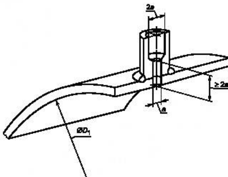
Рисунок А.1 — Конструкция приемника статического давления
