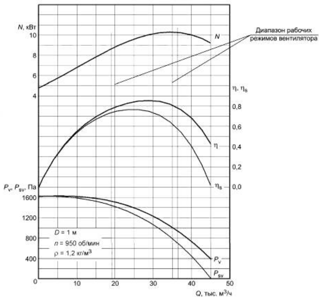
Рисунок Ж.1 — Размерные аэродинамические характеристики радиального вентилятора
