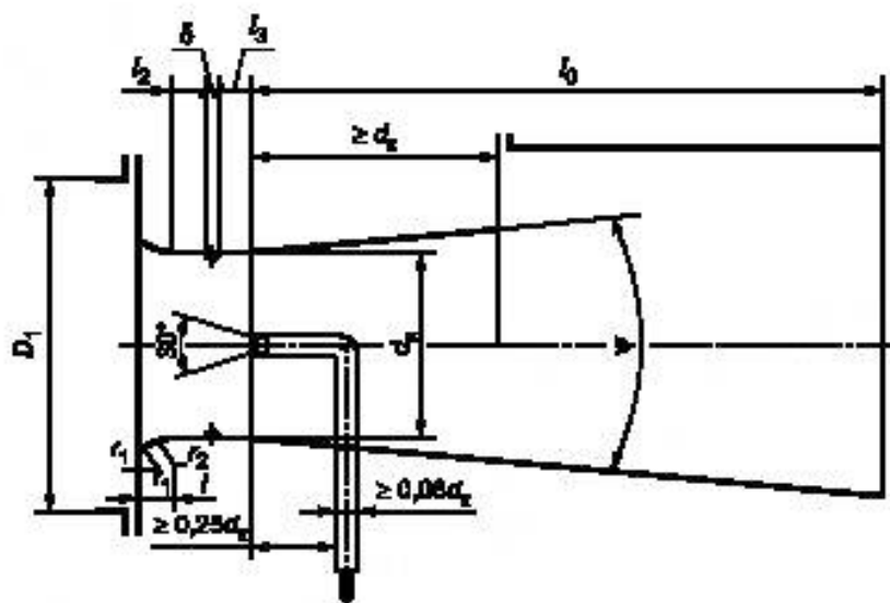
Рисунок В.3 — Геометрические размеры встроенного сопла Вентури
