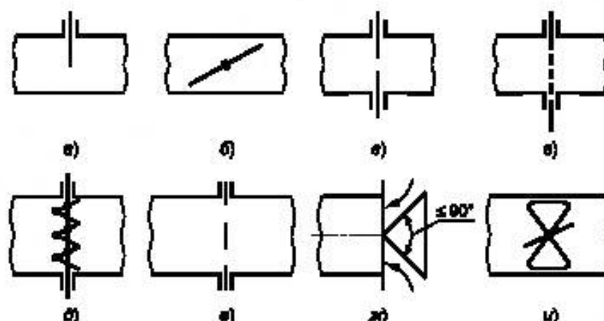
Рисунок 6 — Схемы дросселирующих устройств
