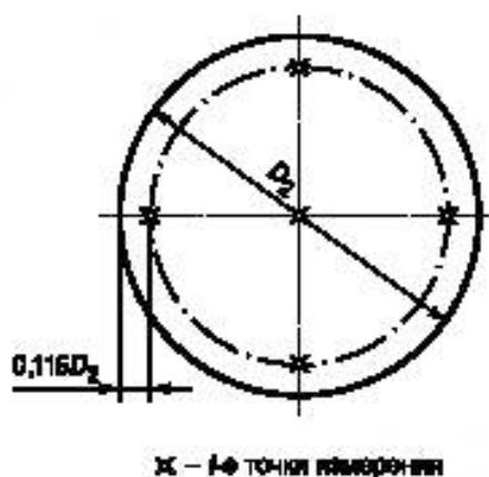
Рисунок Д.1 — Схема измерений полных давлений
