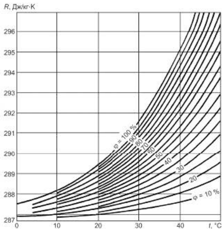
Рисунок Е.2 — Зависимость газовой постоянной R от температуры t и относительной влажности \varphi_{\text{в}}
