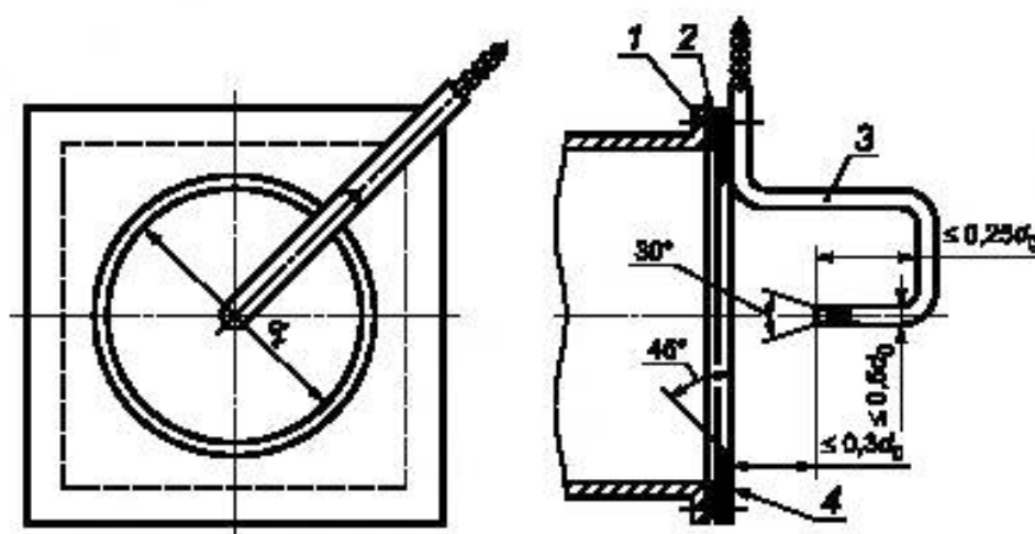
1 — выходной патрубок вентилятора; 2 — диафрагма; 3 — приемник полного давления (трубка Пито); 4 — резиновая прокладка
