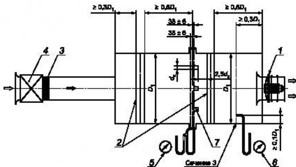
1 — испытуемый вентилятор; 2 — устройства выравнивания потока; 3 — струеуспокоитель; 4 — вспомогательный вентилятор; 5 — дифференциальный манометр для измерения разности давлений в расходомере; 6 — приемник полного давления для измерения давления; 7 — сопло
