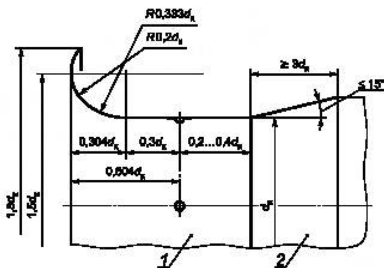
Рисунок В.2 — Входное сопло Вентури (двухрадиусное)
