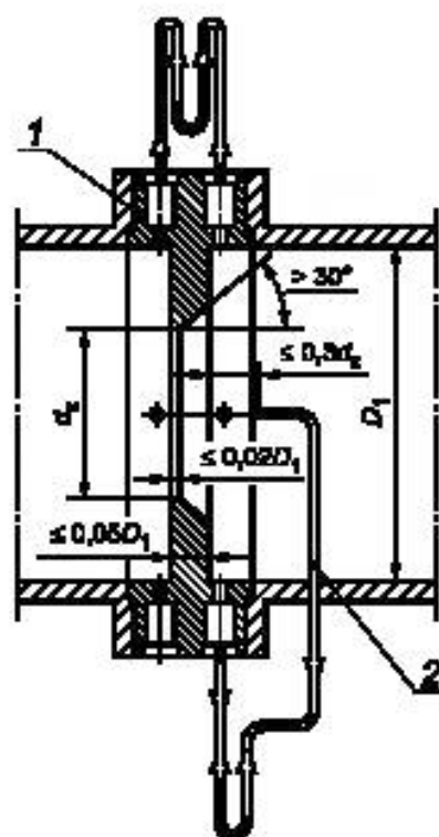
1 — диафрагма; 2 — трубка Пито
