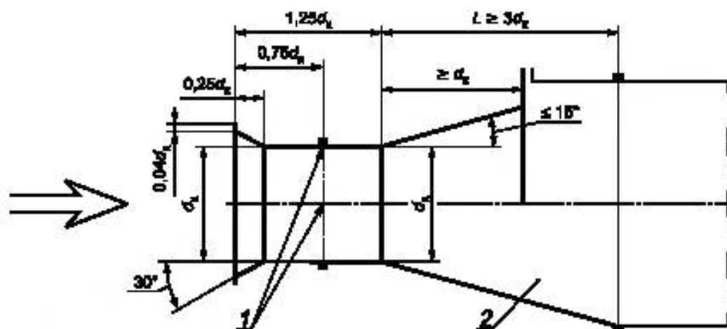
Рисунок В.1 — Конический входной коллектор
