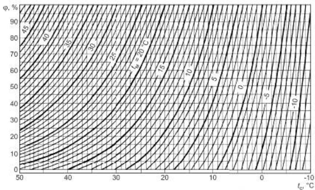
Рисунок Е.1 — График для определения относительной влажности воздуха \varphi_s по показателям сухого и мокрого термометров
