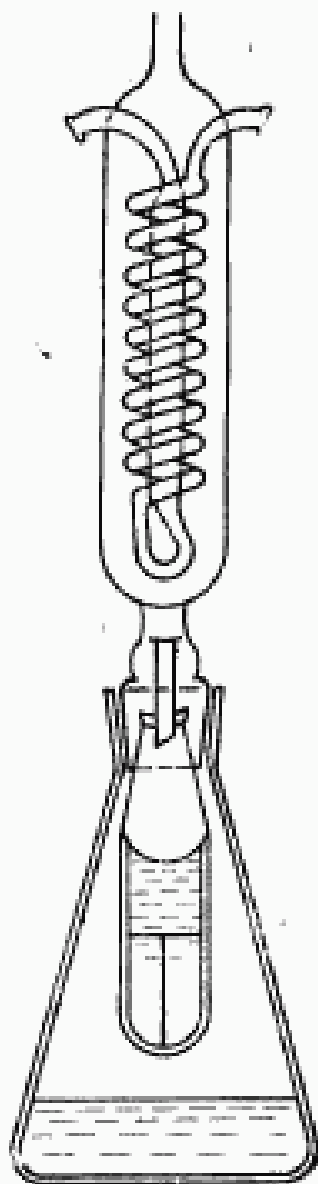
Аппарат для определения выхода толуольного экстракта
