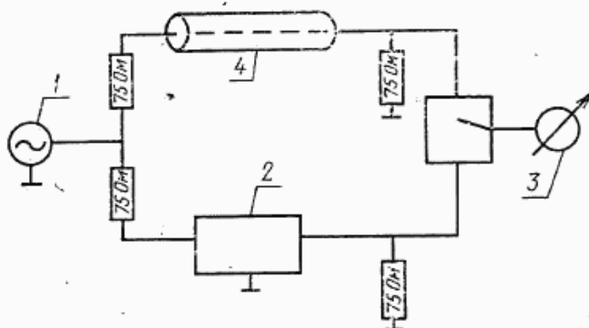
1—генератор; 2—магазин затухания; 3—индикатор; 4—измеряемая коаксиальная линия
