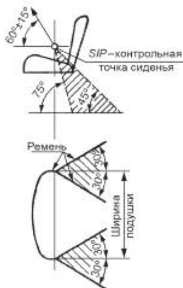
Рисунок Б.1 — Места крепления ремней безопасности
