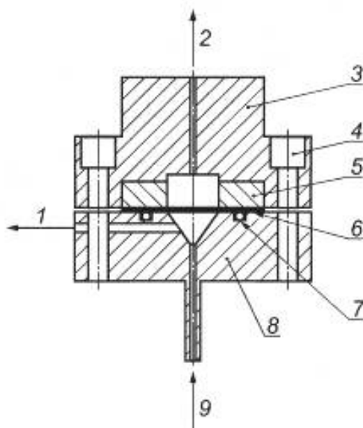
Рисунок 1 — Испытание диска
