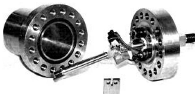
Рисунок 7 — Камера из нержавеющей стали с загрузочными штангами и образцом
