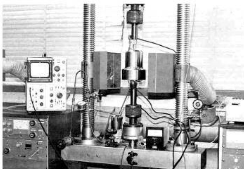
Рисунок 8 — Сервогидравлическая установка для испытаний
