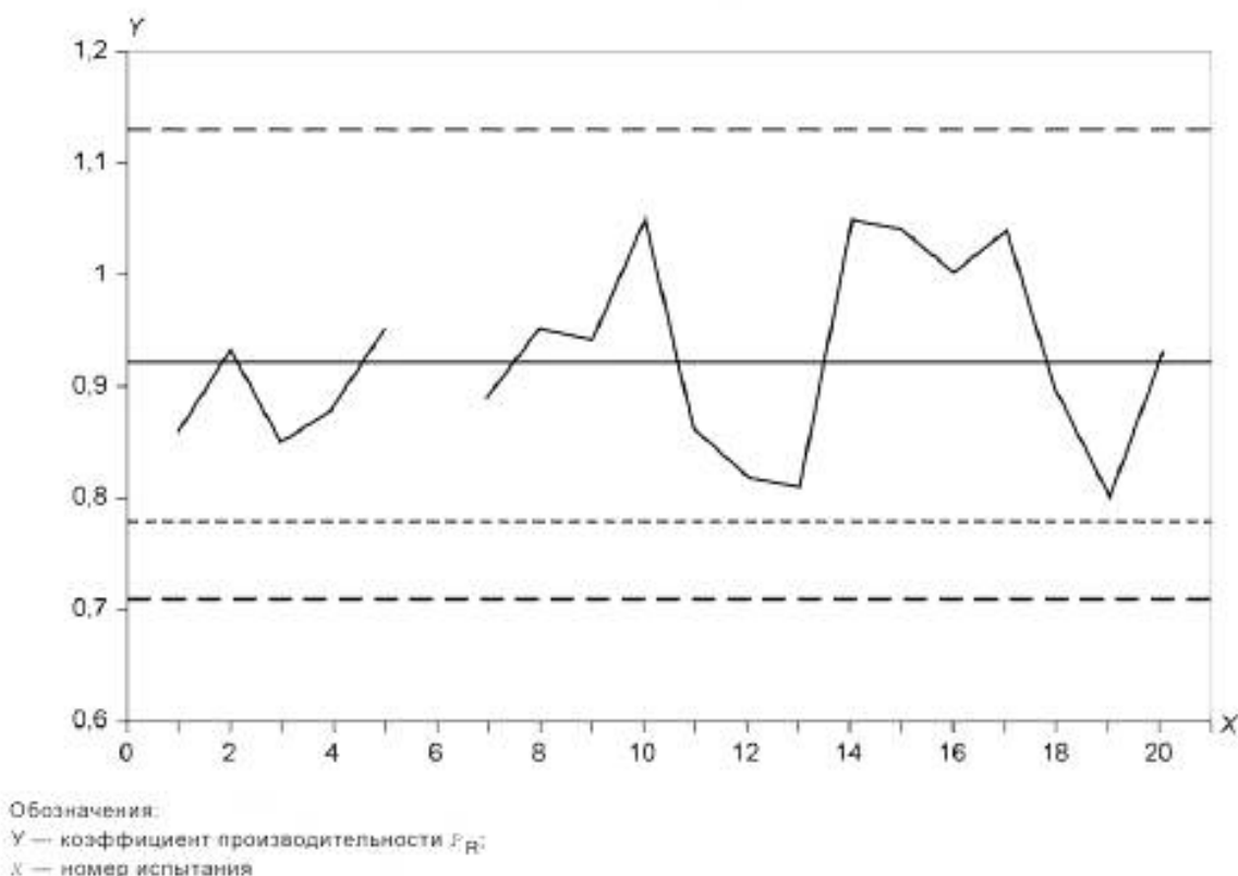
Рисунок G.1 — Контрольный график, составленный на основе значений коэффициента производительности, полученных в результате первых 20 проверок, приведенных в таблице G.1 (результат испытания 6, являющийся резко отклоняющимся значением, исключен)
