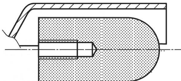
Рисунок 13 — Защитное ограждение абразивных инструментов типов 16, 18, 18R и 19
