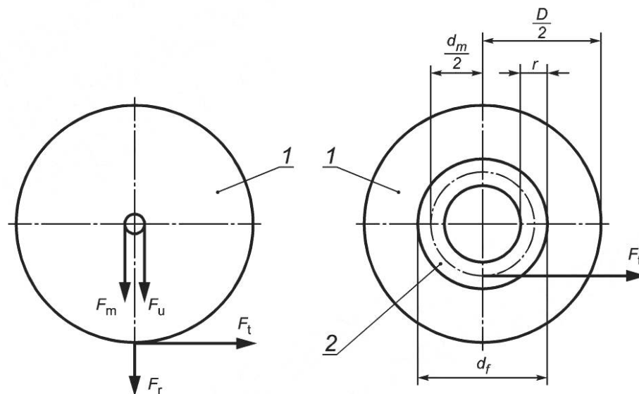
1 — шлифовальный круг; 2 — зажимная кромка фланца
