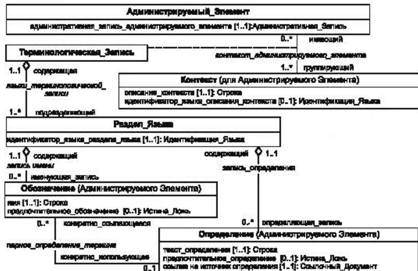
Рисунок 6 — Область Наименования и Определения метамодели (Cor.1:2004)
