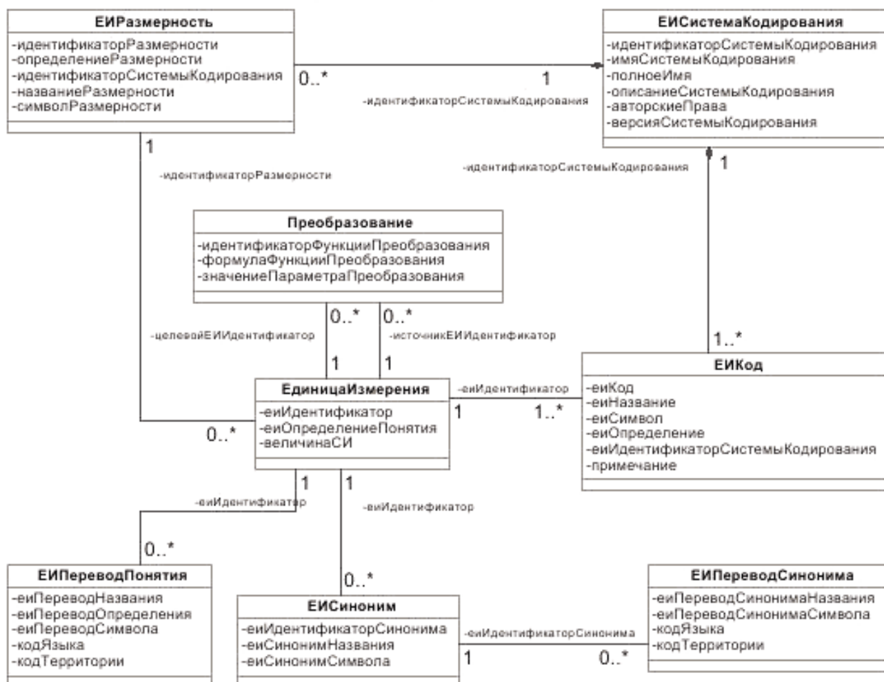
Рисунок 2 – Диаграмма классов UML для понятий единиц измерения
