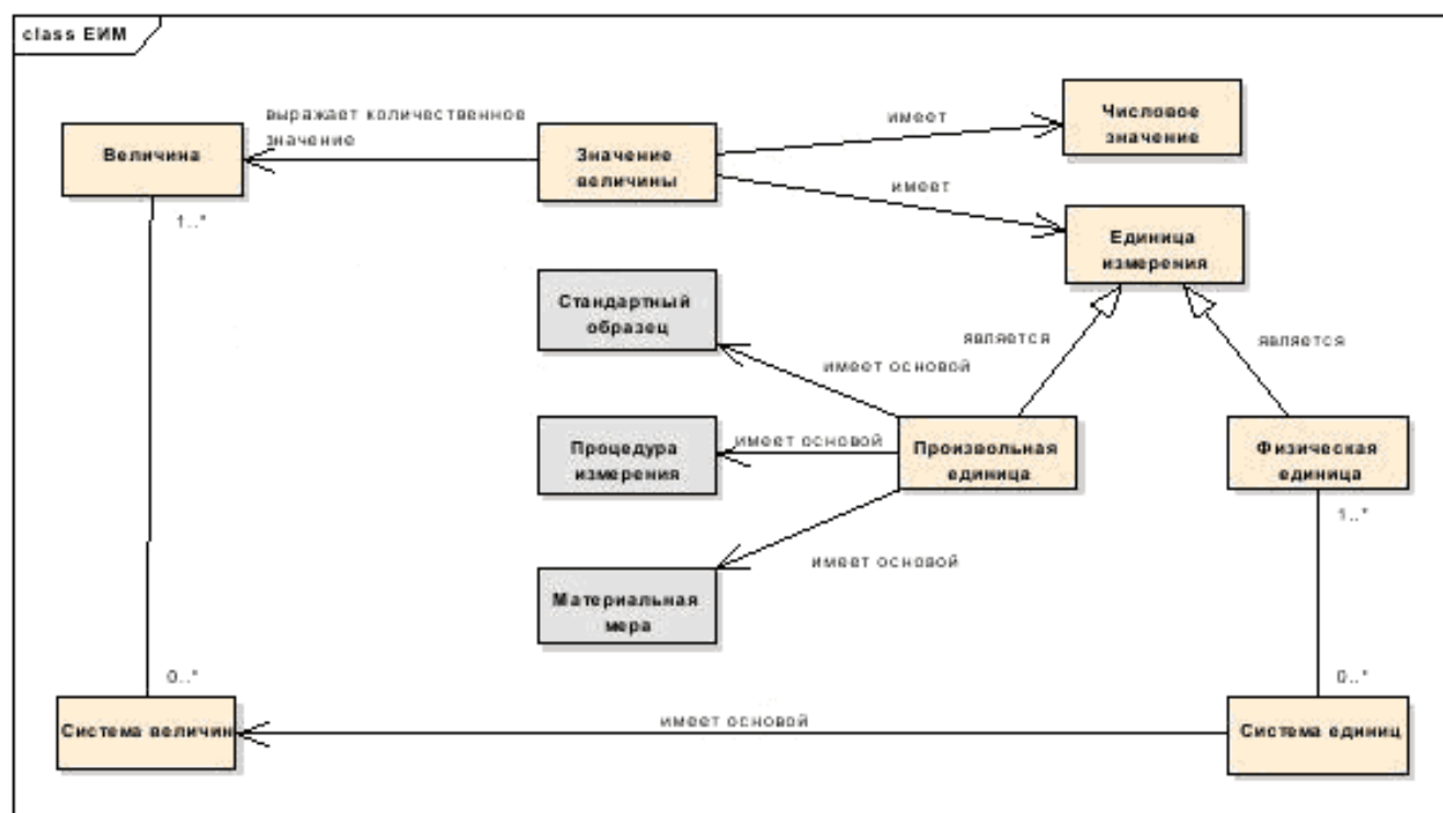
Рисунок 1 – Схематическая концептуальная модель единиц измерения и связанных понятий, приведенных в разделе 3, в виде диаграммы классов на языке UML
