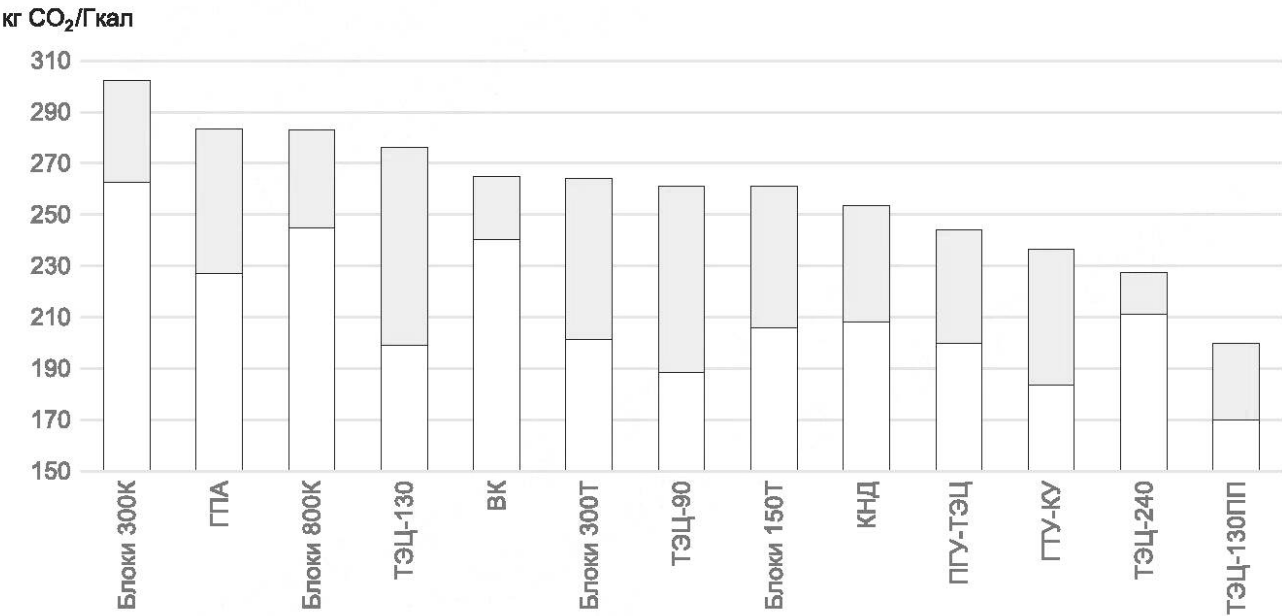
Рисунок Б.1 — Интервалы среднегодовых значений удельных выбросов ПГ на единицу отпущенной тепловой энергии при работе КТЭУ на газообразном топливе
