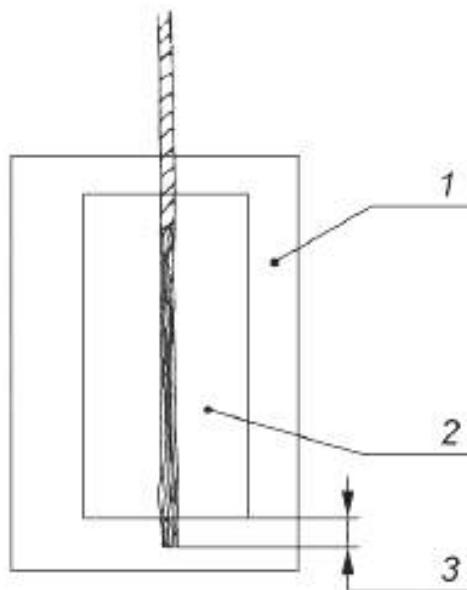
1 — бархатные доски; 2 — стеклянная тарелка; 3 — примерно 5 мм
