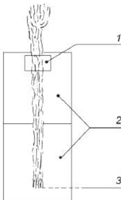
1 — взвешенная стеклянная пластина; 2 — бархатные доски; 3 — выровненный конец
