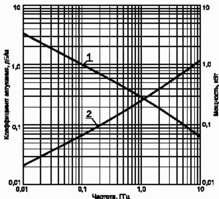
Частотные зависимости
