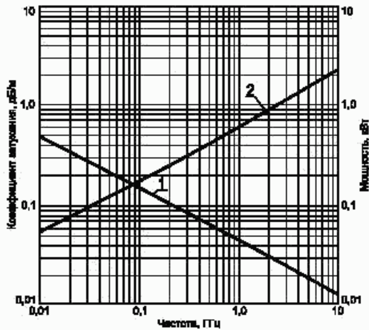
Частотные зависимости
