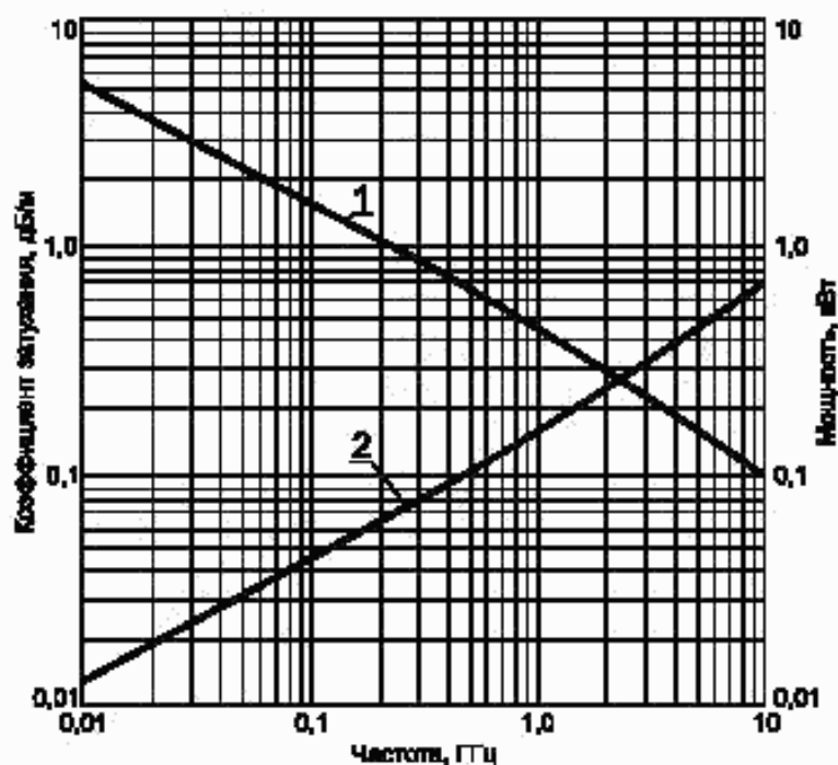
Частотные зависимости
