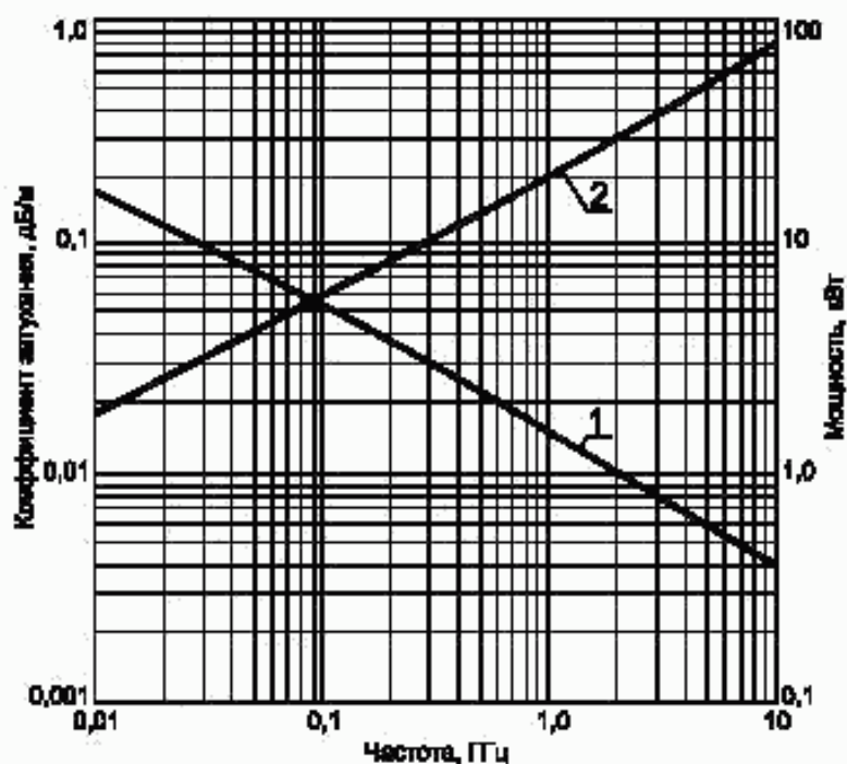
Частотные зависимости
