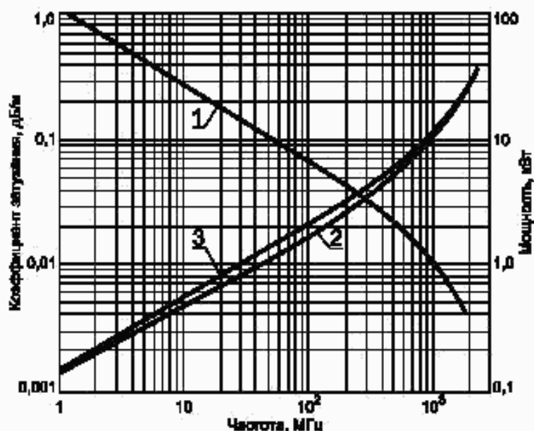
Частотные зависимости
