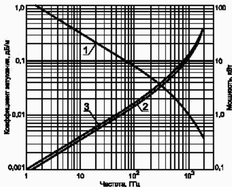
Частотные зависимости
