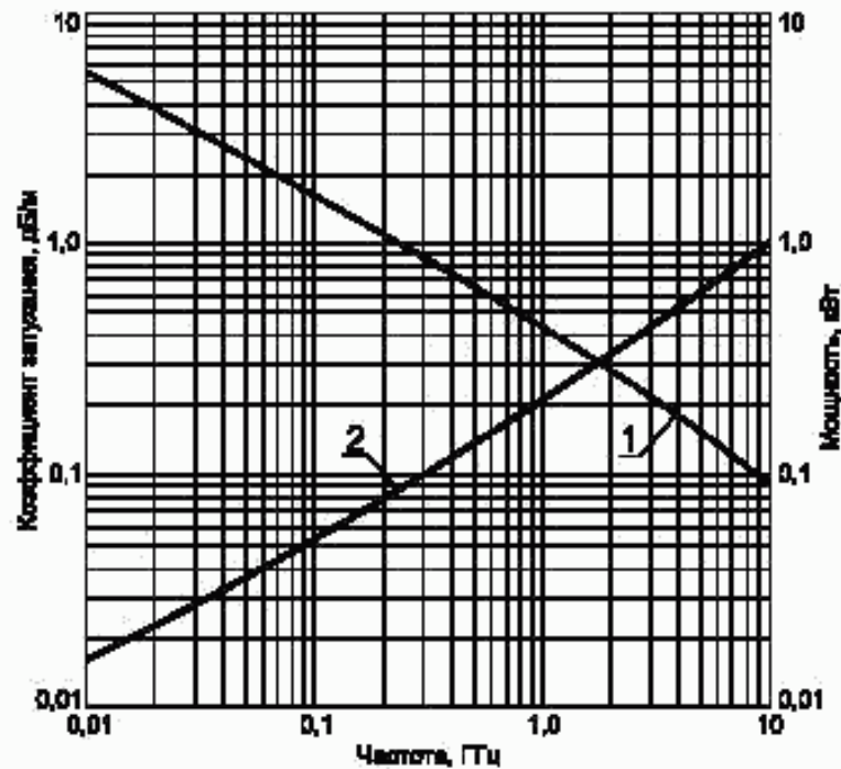
Частотные зависимости
