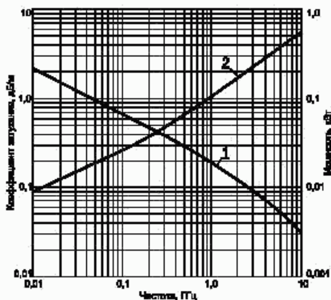
Частотные зависимости
