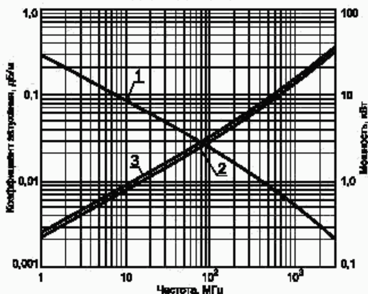
Частотные зависимости
