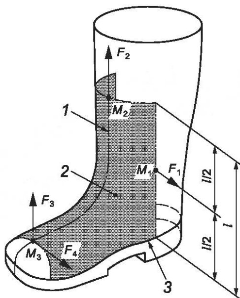
Рисунок 3 — Место испытания и направления для испытания на растяжение
