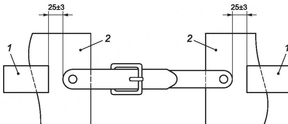
1 — зажим; 2 — гетра
