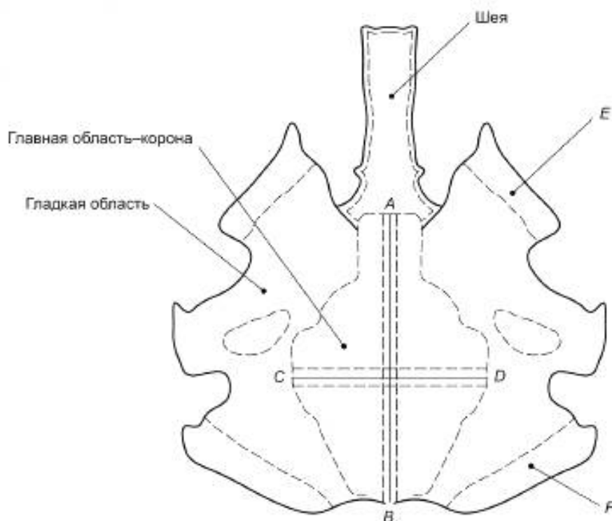
Рисунок 1 — Кожа страуса
