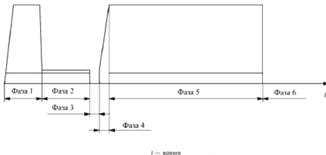
Рисунок А.1 — Цикл сварки встык
