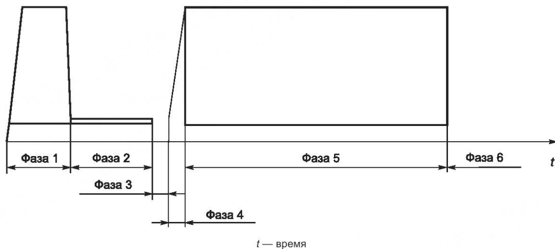
Рисунок А.1 — Цикл сварки нагретым инструментом встык
