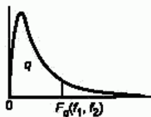
Рисунок 1 — Квантили F-распределения
