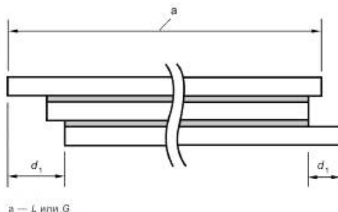
Рисунок 5 — Смещение листов стекла в моллированном многослойном стекле
