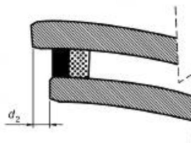
Рисунок 7 — Смещение стекол в моллированном стеклопакете
