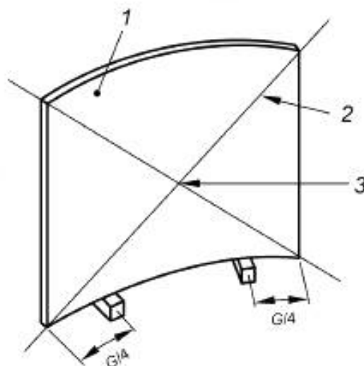
Рисунок 10 — Измерение максимально допустимого перекося
