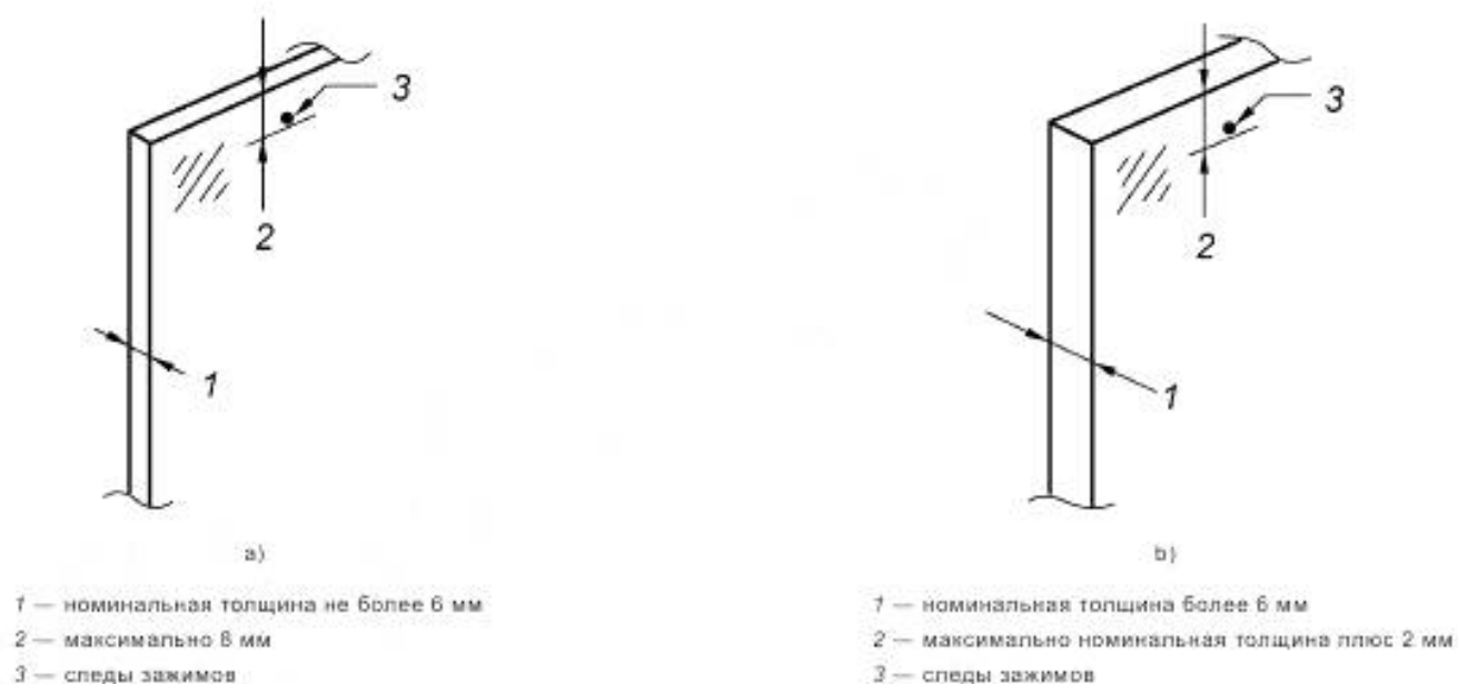
Рисунок 4 — Следы зажимов
