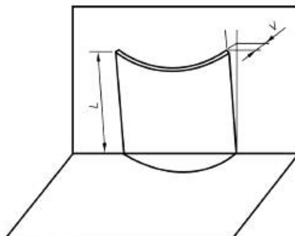
Рисунок 3 — Допустимый перекосяк
