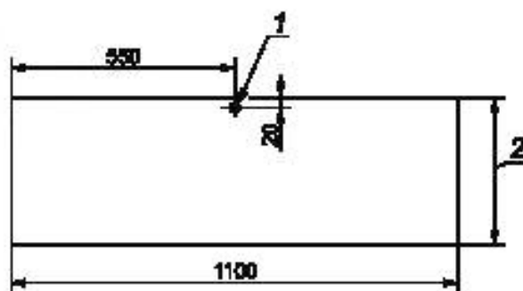
1 — точка удара; 2 — ширина образца 360 или 500 мм
