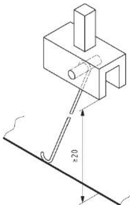
Рисунок 2 — Захватывающий крюк
