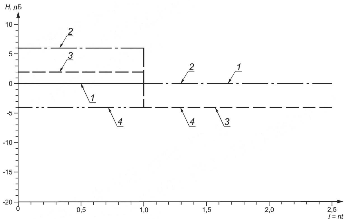
Рисунок А.5 — Уровень приемки 2 (AL 2). Уровни при применении способа 2 для контроля толщин от 8 до 15 мм
