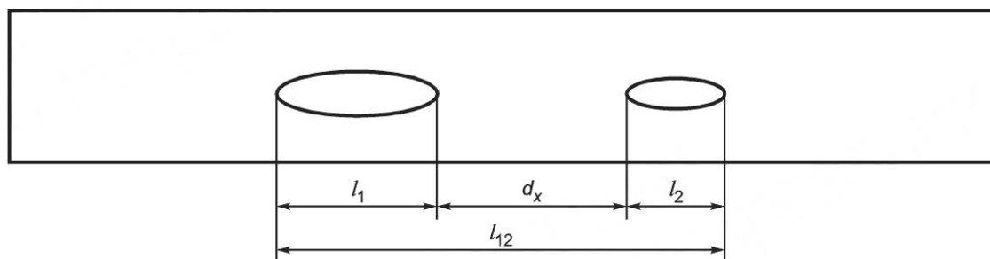
Рисунок 1 — Геометрическая конфигурация для сгруппированных несплошностей
