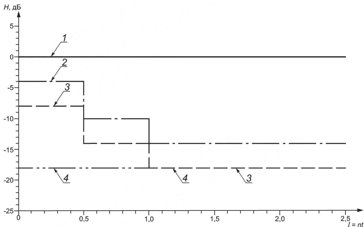
Рисунок А.9 — Уровень приемки 3 (AL 3). Уровни при применении способа 2 для контроля толщин от 15 до 100 мм
