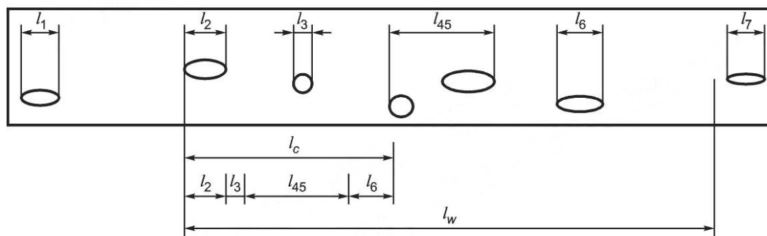
Рисунок 3 — Суммарная протяженность несплошностей
