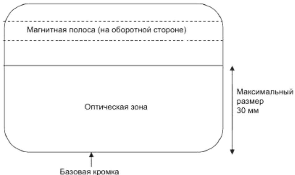
Рисунок 2 – Карта с магнитной полосой
