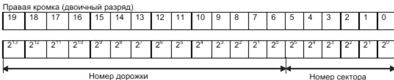
Рисунок 4 – Формат адреса сектора и дорожки
