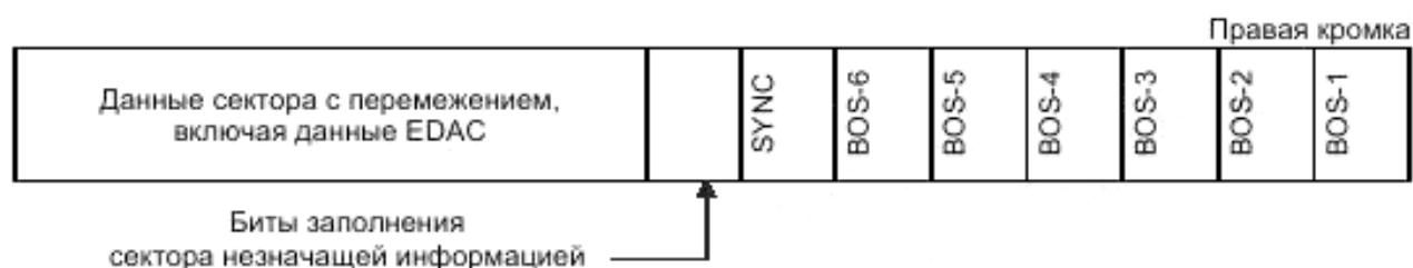
Рисунок 8 – Структура сектора, типы 0 – 5
