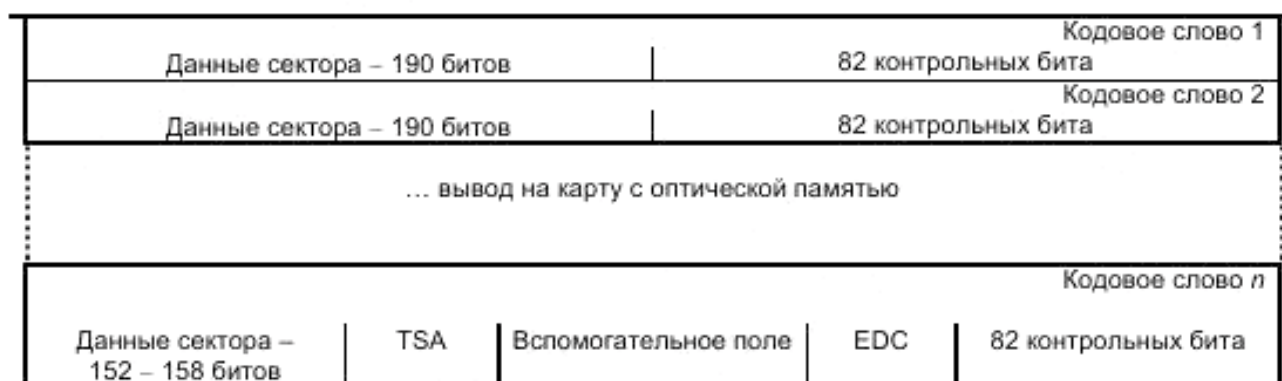
Рисунок 13 – Перемежевание данных сектора с кодом EDAC, секторы типов 0 – 4
