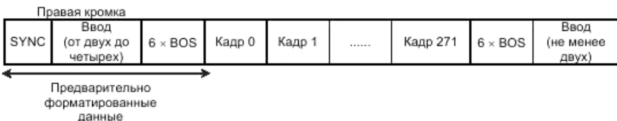
Рисунок 7 – Структура дорожки (с полной и частичной записью) для секторов с максимальным перемерением, типы 7 – 15
