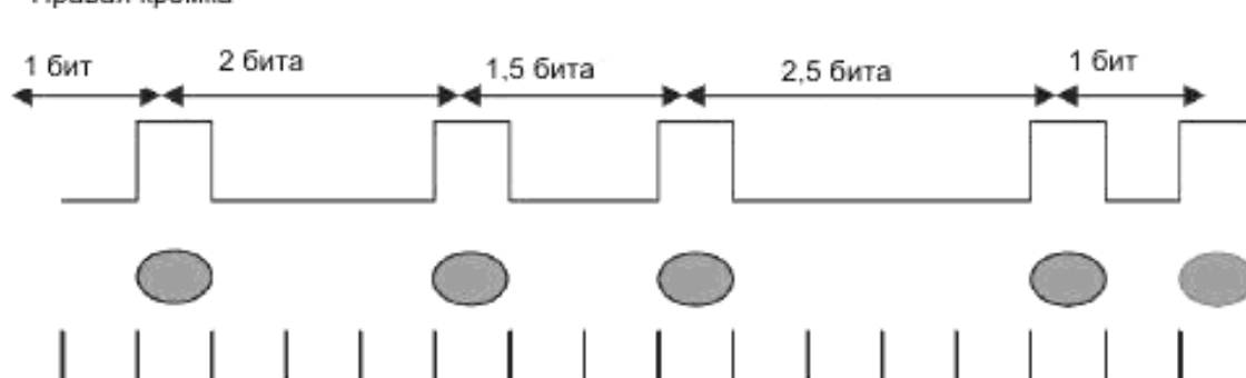
Рисунок 2 – Структура синхронизирующей метки
