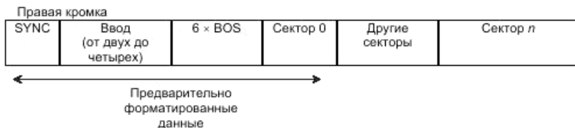
Рисунок 6 – Структура дорожки с неполной записью, секторы типов 0 – 5
