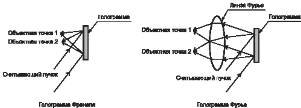
Рисунок А.4 — Голограммы Френеля и Фурье
