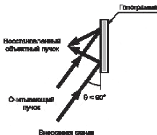
Рисунок А.3 — Осевая и внеосевая схемы голограмм
