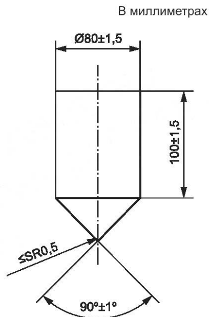
Рисунок 6 — Испытательный конус
