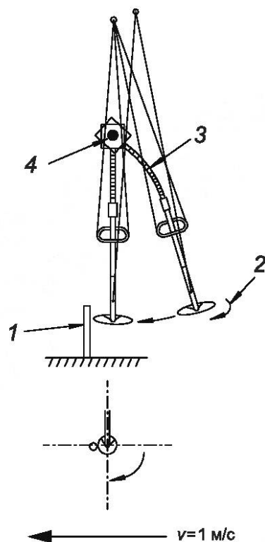
b) Машина с рачевым источником питания
