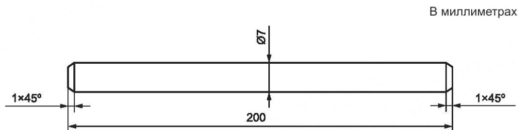
Рисунок Е.1 — Испытательный щуп для определения прочности и доступности топливоподводов
