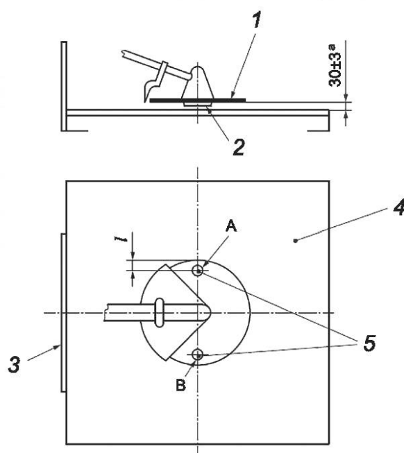
Рисунок В.2 — Положения вставки испытываемых образцов
