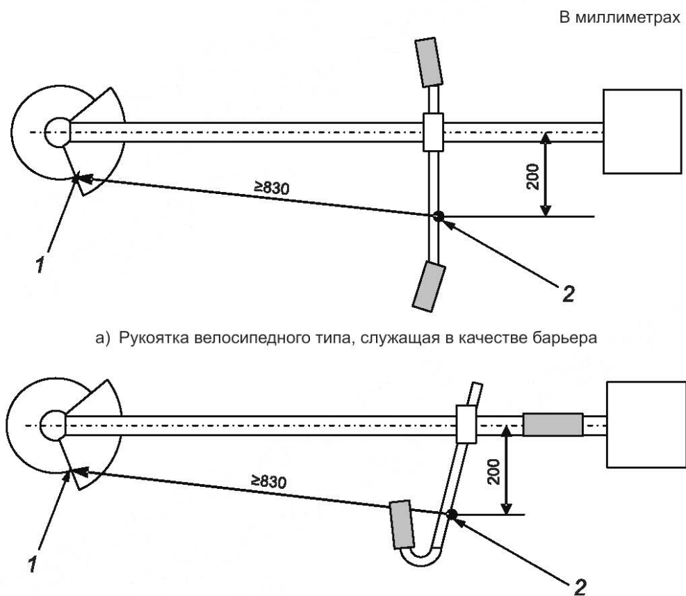
Рисунок 4 — Пример машин с различной конфигурацией рукояток, барьером и расстоянием до режущего инструмента
