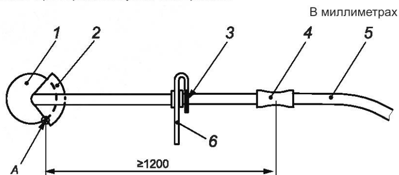
Рисунок 2 — Расстояние до режущего инструмента
