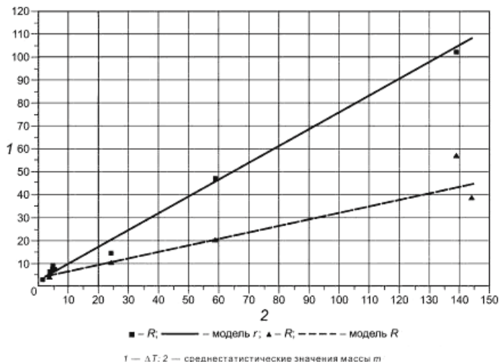
Рисунок А.1 — Статистическая модель для \Delta T , °C
