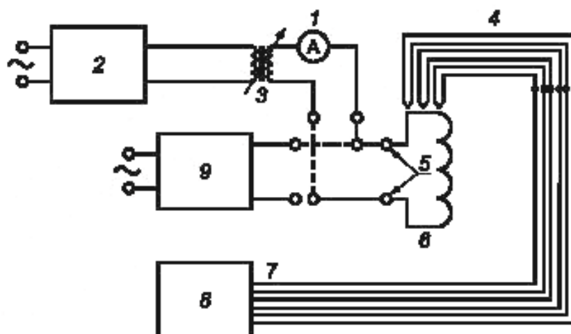
Рисунок 4 — Схема расположения основного и дополнительного оборудования
