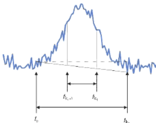
Рисунок 4 – Модели наложения выше горизонтальной линии (пунктирная линия) и наклонной линии (сплошная линия) между точками t_{k_c+1} и t_{k_c}
