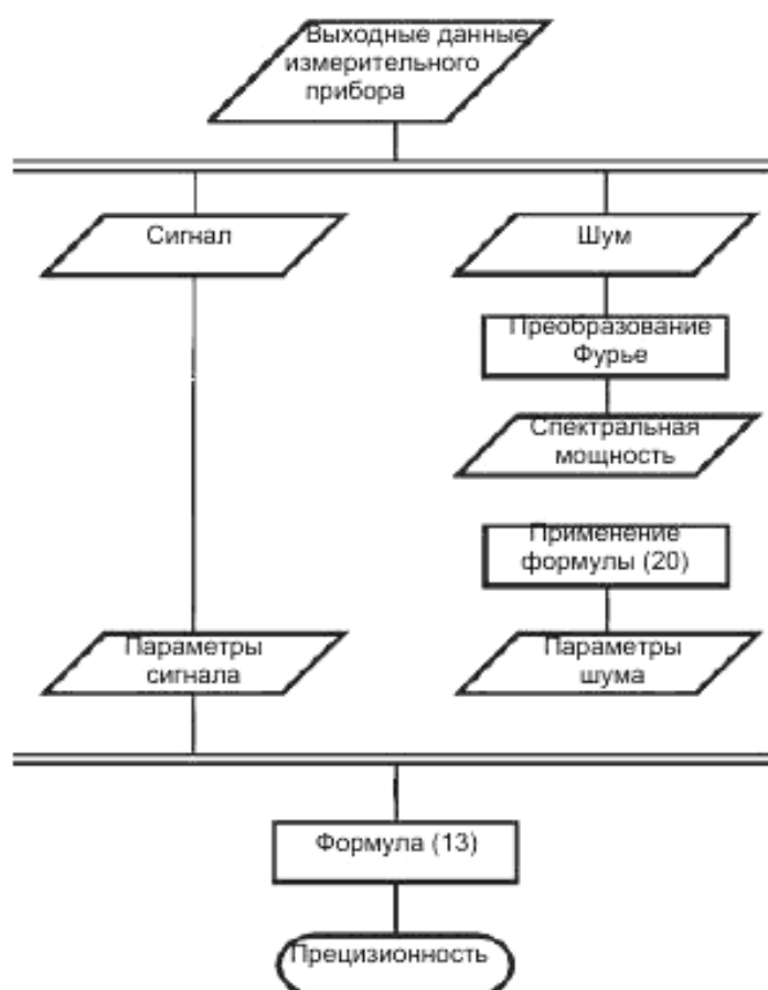
Рисунок 6 – Процедуры теории FUMI
