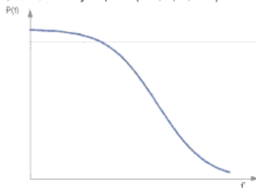
Рисунок 5 – Спектральная плотность мощности смоделированного шума
