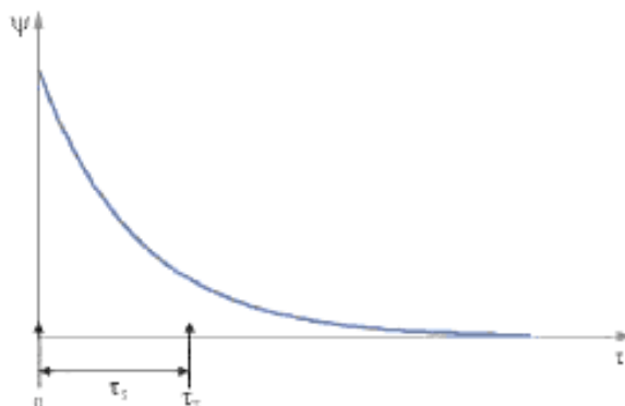
Рисунок 2 – Функция автоковариации шума
