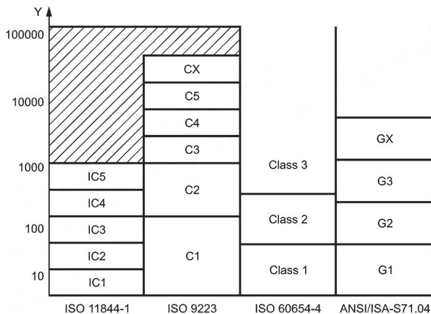
Рисунок А.2 — Классификация коррозионной агрессивности меди в соответствии с ISO, IEC и ISA
