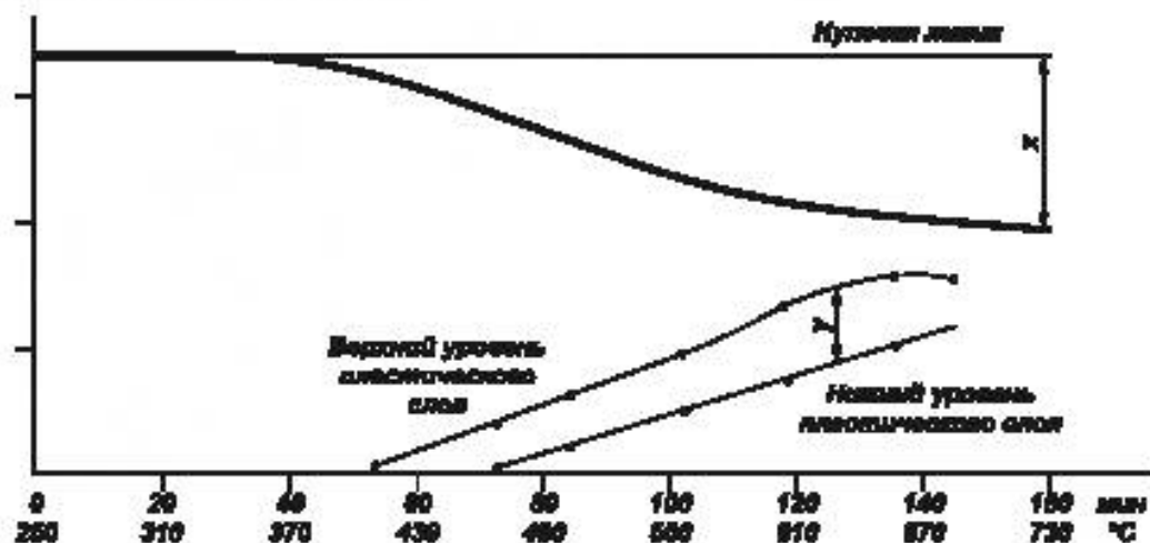
Рисунок 6 — Пологопадающая кривая
