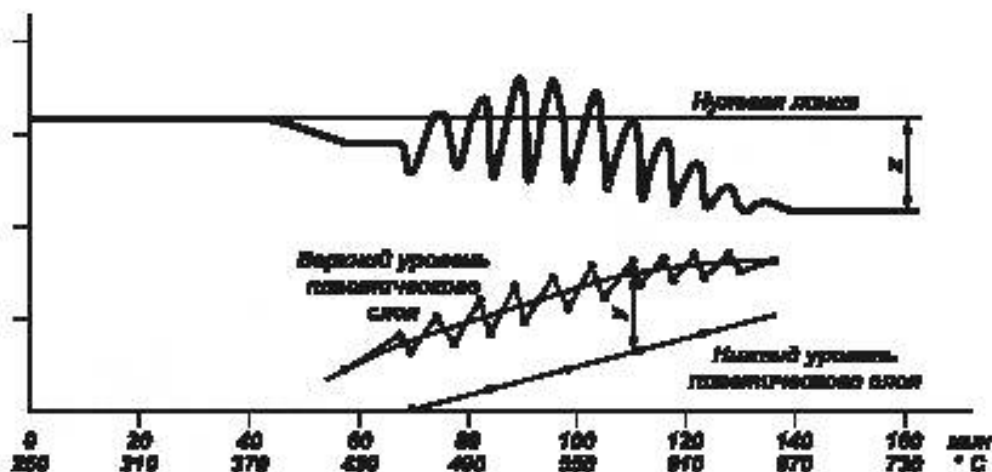
Рисунок 8 — Зигзагообразная кривая
