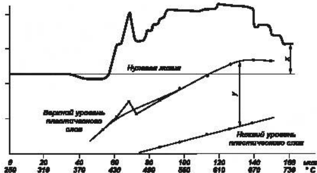
Рисунок 7 — Горбообразная кривая с отрицательной усадкой
