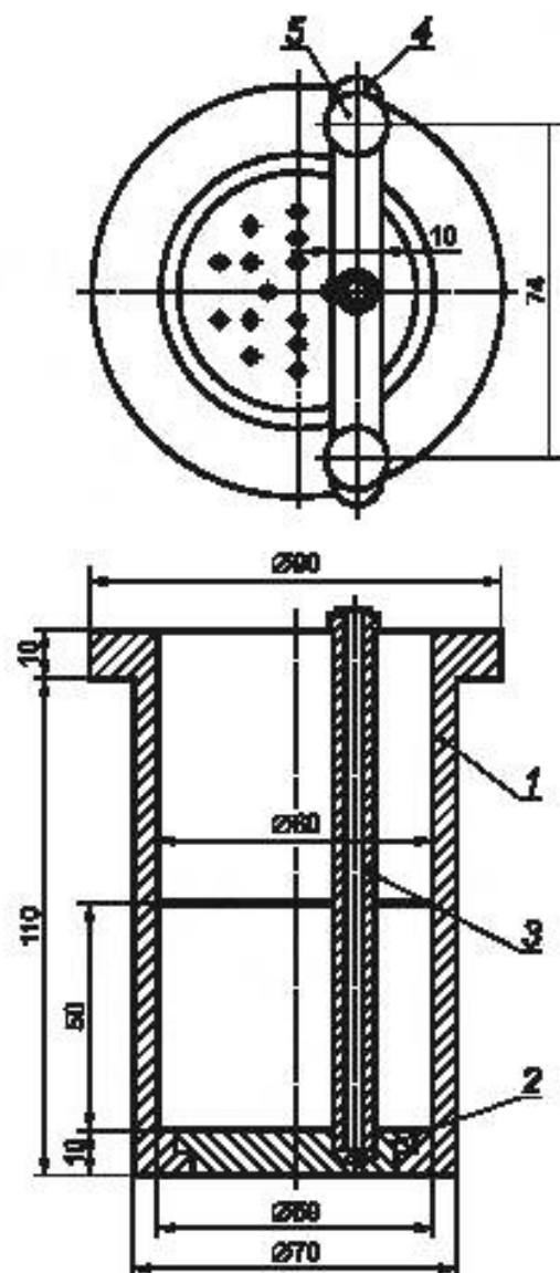
1 — корпус; 2 — доньшко; 3 — трубка для термопары; 4 — прижимная планка; 5 — прижимной винт
