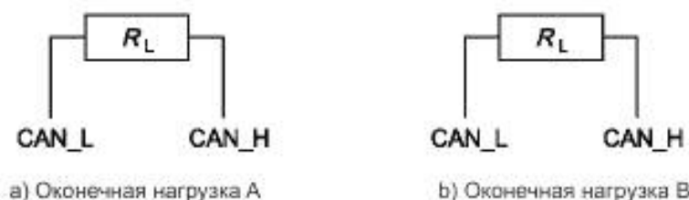
Рисунок 14 — Оконечная нагрузка для высокоскоростной реализации шины
