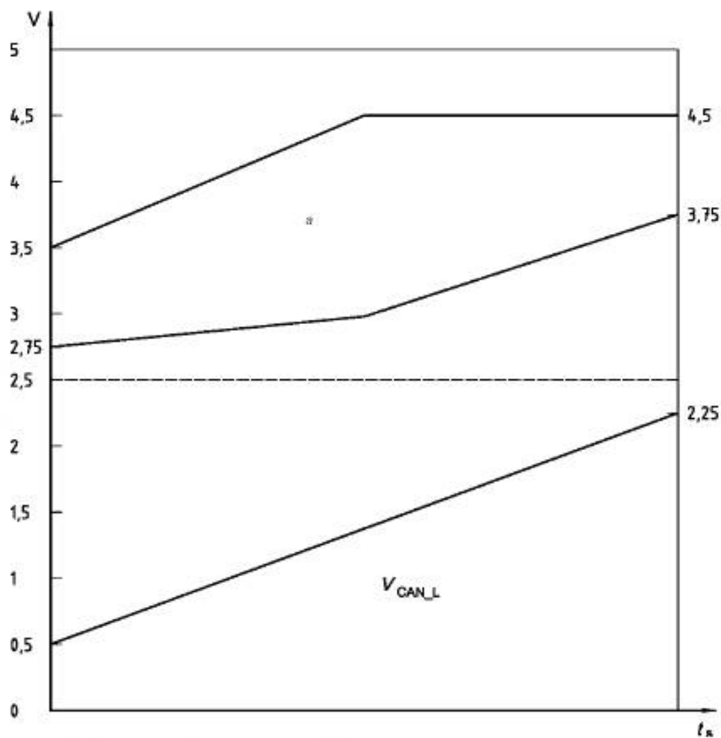
Рисунок 17 — Допустимые диапазоны напряжения V_{CAN\_H} при доминантном состоянии узла CAN, отключенного от шины, и при изменении V_{CAN\_L} от минимального до максимального уровня напряжения
