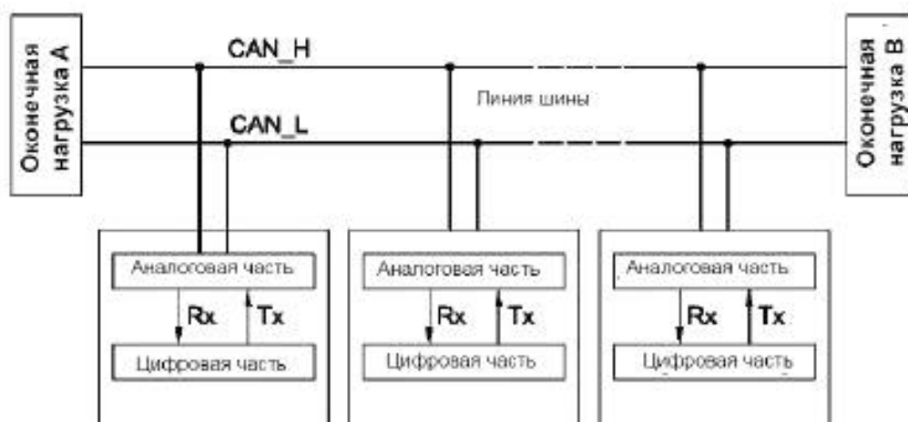
Рисунок 1 — Рекомендуемое электрическое подключение
