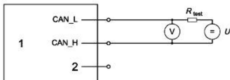
1 — узел CAN со схемой оконечной нагрузки; 2 — заземление
