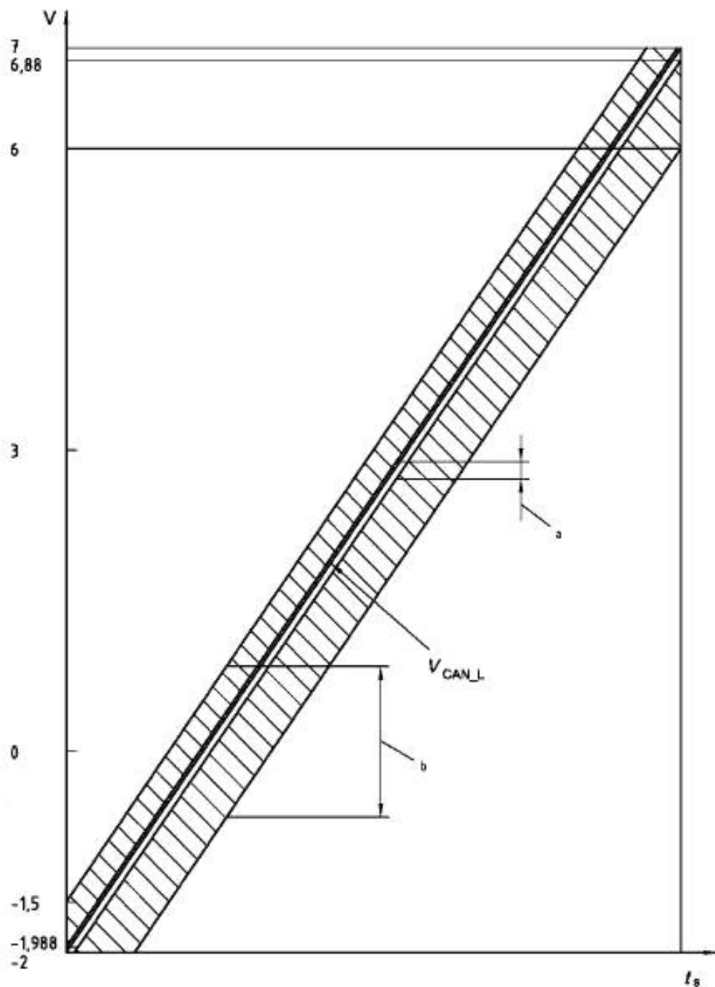
Рисунок 16 — Допустимые диапазоны напряжения V_{CAN\_H} для мониторинга рецессивного состояния шины при отключении узла CAN и изменении V_{CAN\_L} от минимального до максимального уровня синфазного напряжения на шине
