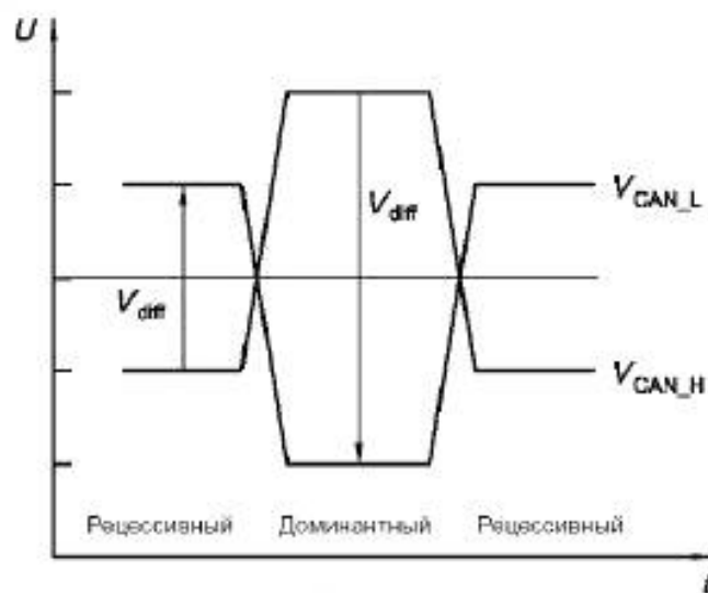
Рисунок 2 — Физическое представление битов
