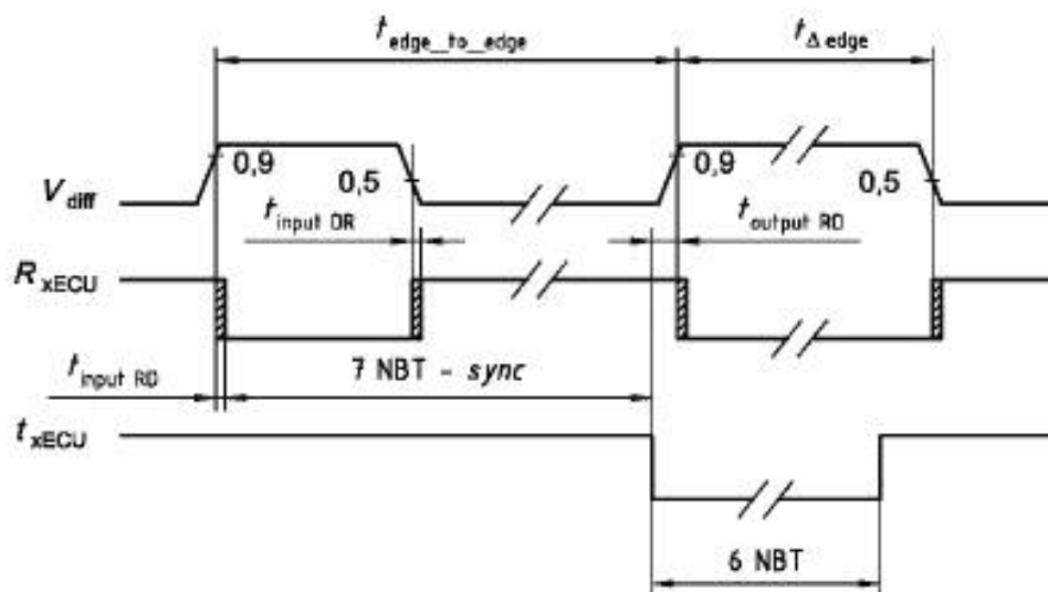
Рисунок 12 — Измерение времени внутренней задержки ECU
