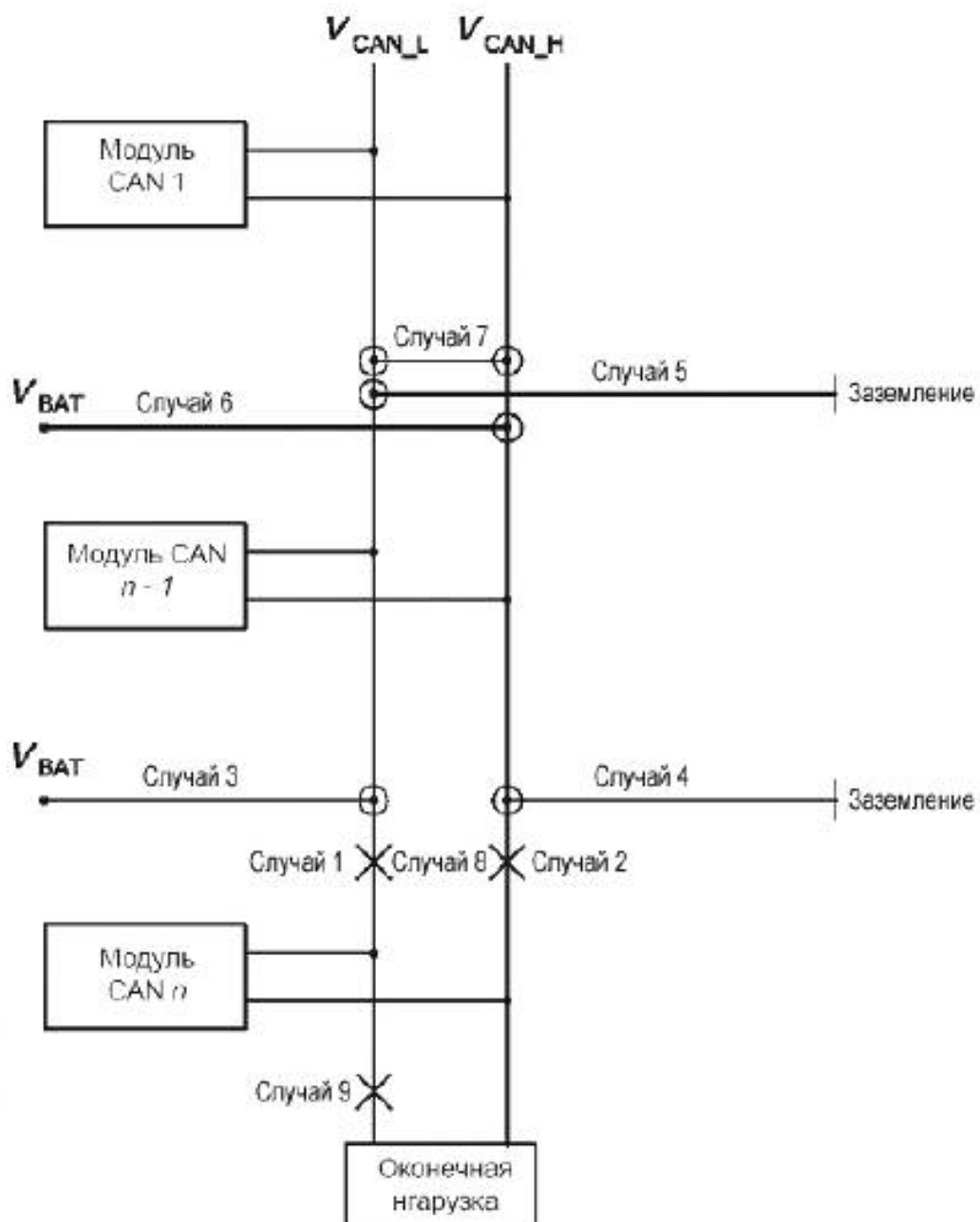
Рисунок 19 — Возможные отказы линий шины
