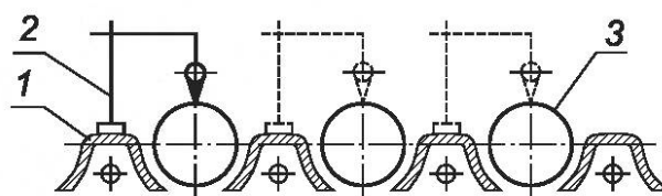
1 — верхний блок станка; 2 — средство измерений; 3 — валец
