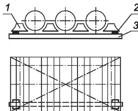
1 — опорная балка; 2 — опоры; 3 — поверочная линейка
