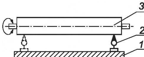
1 — опорная балка; 2 — средство измерений; 3 — подающий валец
