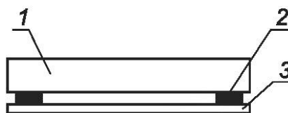
1 — опорная балка; 2 — опоры; 3 — поверочная линейка
