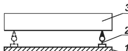
1 — рабочая поверхность конвейера; 2 — средство измерений; 3 — опорная балка
