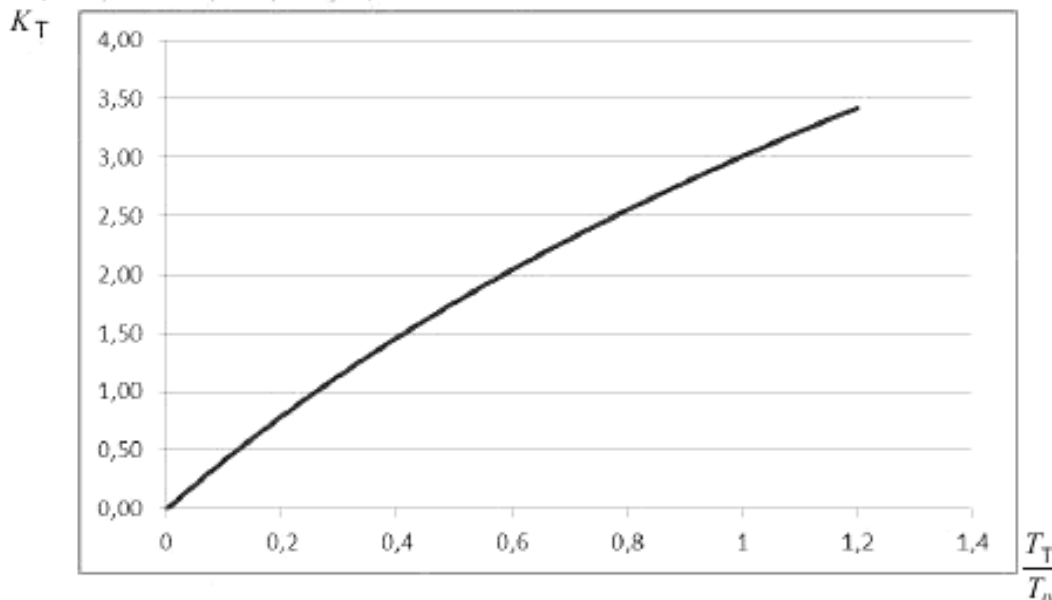
Рисунок А.1 – Зависимость K_T , дБ, от T_T/T_0
