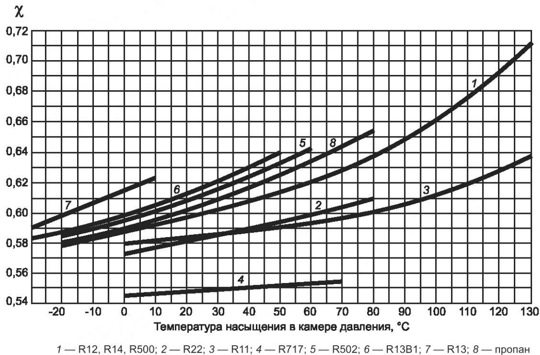
Р и с у н о к Б.3 — Значение коэффициента \chi для критического давления потока.
