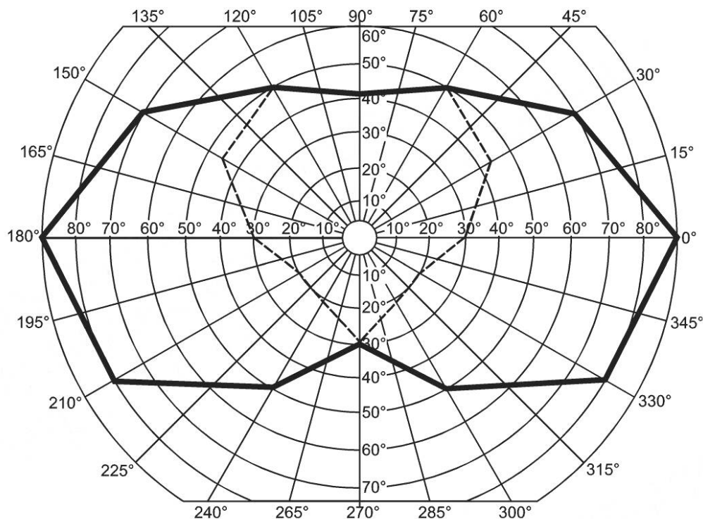
б) Пример диаграммы, получаемой по результатам испытаний (см. 6.3.5—6.3.7)
