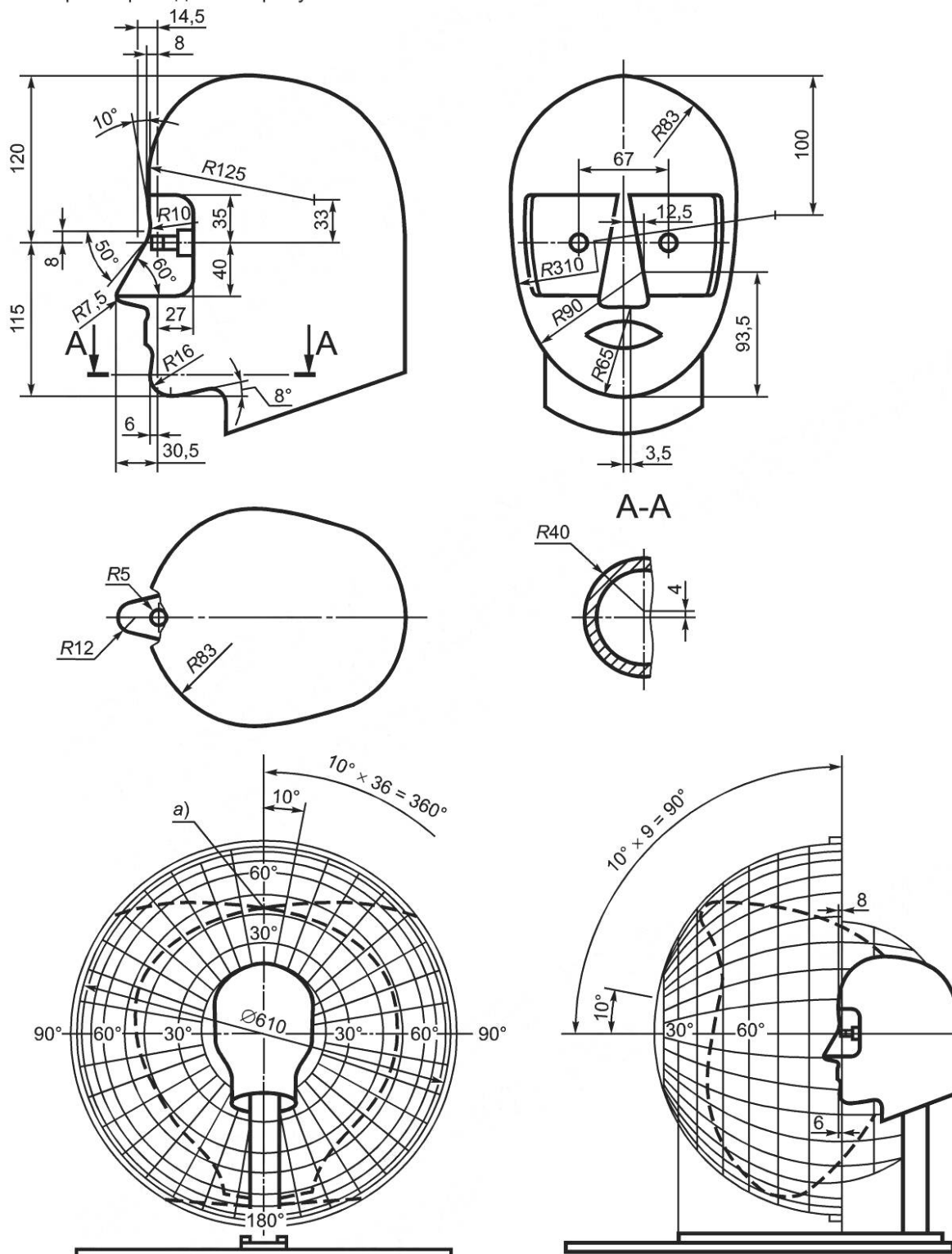
Рисунок 1 — Схема апертометра для определения ограничения поля зрения
