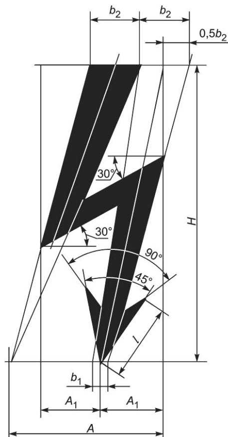
Рисунок Н.1 — Графический символ электрического напряжения
