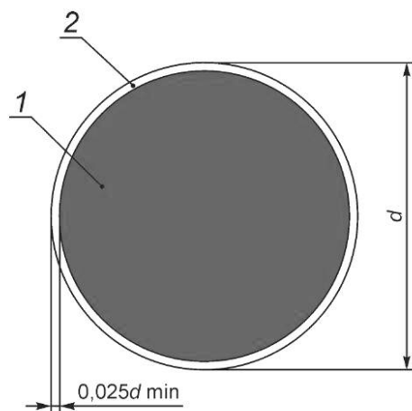
Рисунок 3 — Основа цветографического изображения и соотношение размеров предписывающих знаков безопасности
