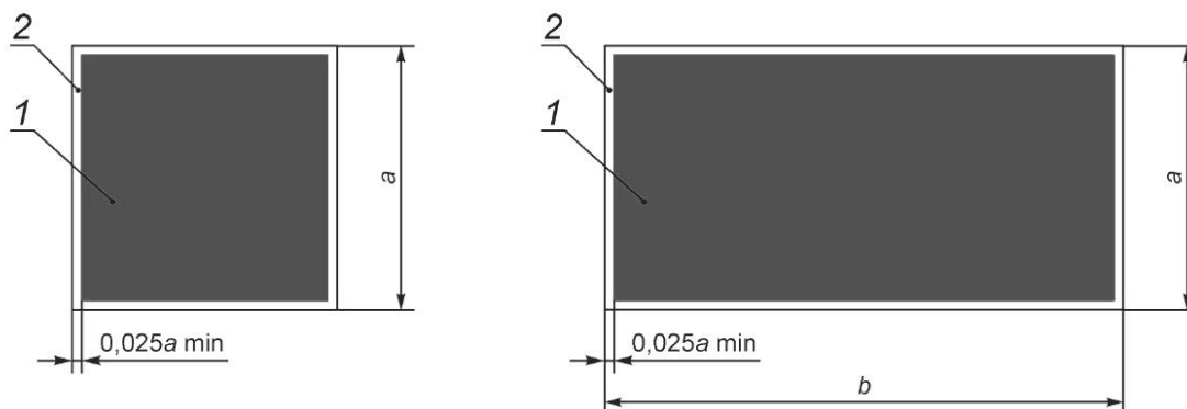
a, b — стороны квадрата и прямоугольника ( 2a = b ); 1 — основная поверхность; 2 — кант
