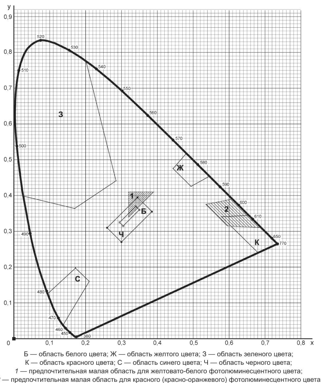
Рисунок Б.1 — Допустимые области цветности сигнальных и контрастных цветов фотолюминесцентных материалов на стандартном цветовом графике x, y МКО 1931 г.
