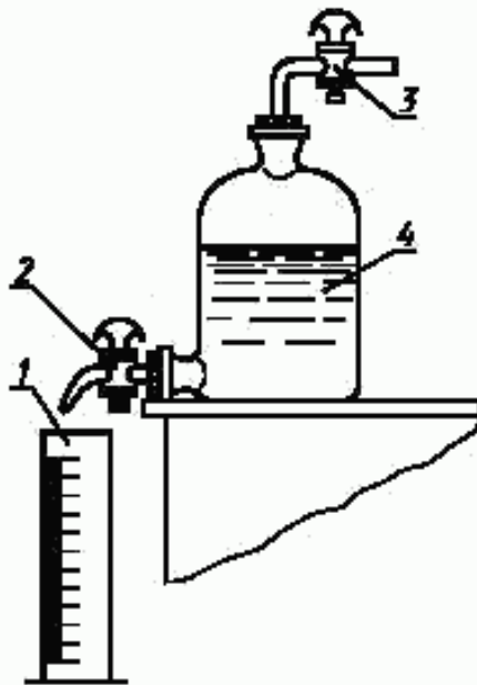
Аспиратор с измерительным цилиндром
