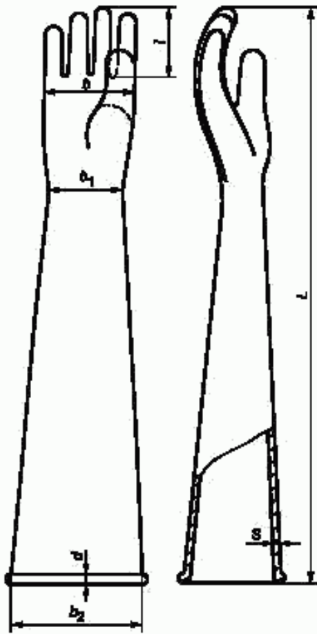
Рисунок Б.1 — Пятипалая перчатка
