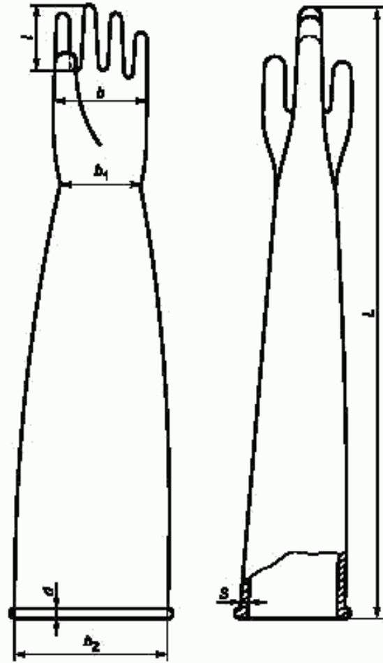
Рисунок Б.2 — Шестипалая перчатка
