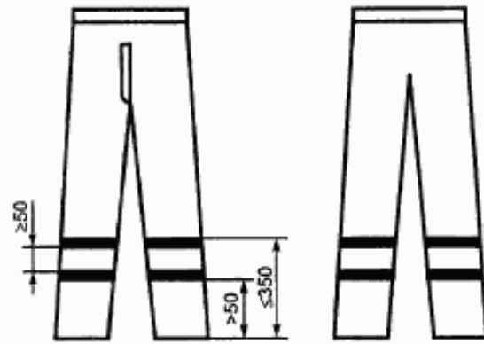
Рисунок Б.9 — Брюки
